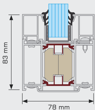
řez pevnou stěnou EI 15, EI 30
