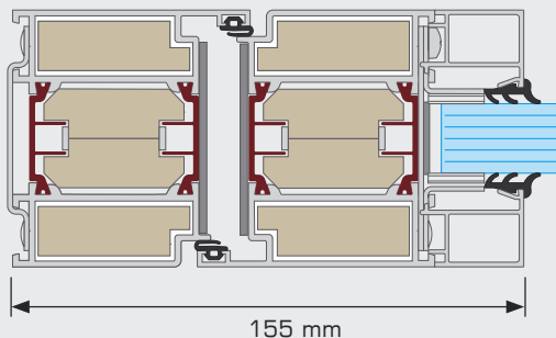
řez dveřmi EI 45, EI 60
